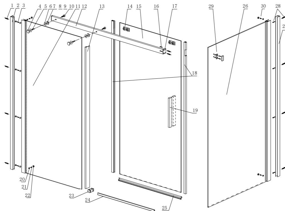
ΠΙΝΑΚΑΣ ΑΝΤΑΛΛΑΚΤΙΚΩΝ / SPARE PARTS CHART / PIÈCES DE TABLE
