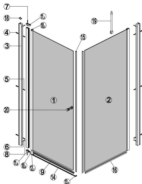
ΠΙΝΑΚΑΣ ΑΝΤΑΛΛΑΚΤΙΚΩΝ / SPARE PARTS CHART / PIÈCES DE TABLE
