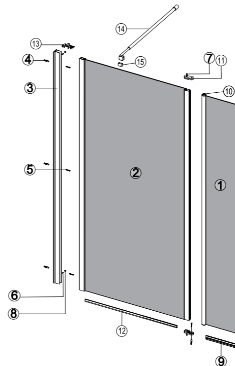
ΠΙΝΑΚΑΣ ΑΝΤΑΛΛΑΚΤΙΚΩΝ / SPARE PARTS CHART / PIÈCES DE TABLE
